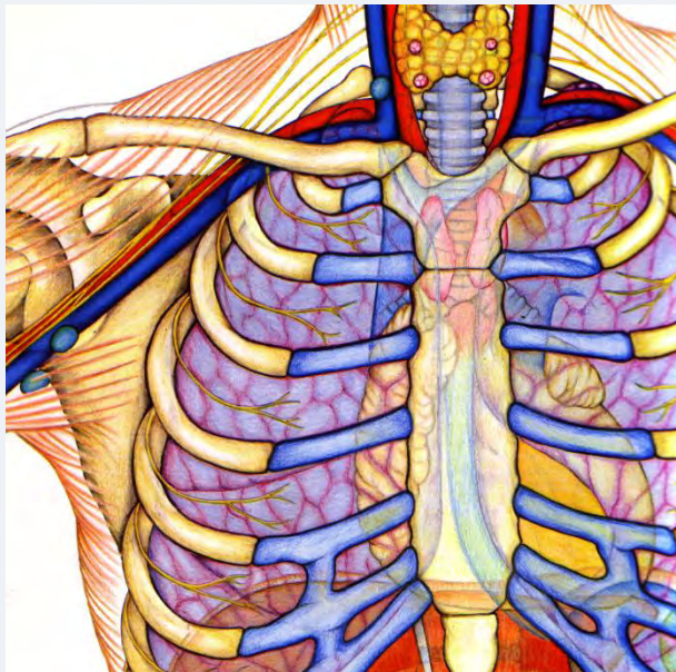
Représentation schématique du médiastin - PJ Wynne
